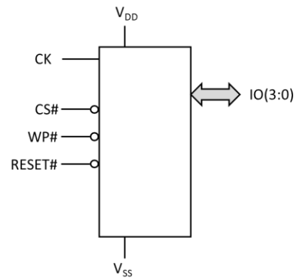
QSPI, DSPI, SPI (8-PIN DFN)
