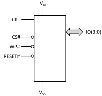
QSPI, DSPI, SPI (8-PIN DFN)
